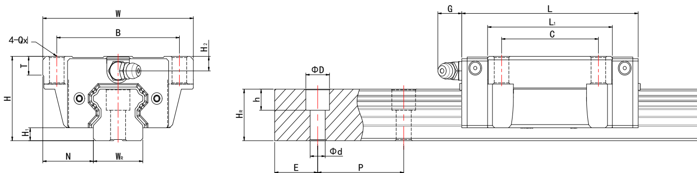
TIWINOK 品牌 11 系列高调心直线导轨 (俗称 HG) 法兰光孔型滑块尺寸表
